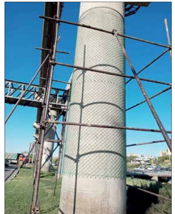
آغاز عملیات اجرای دیوار سبز پایه های منوریل قم
